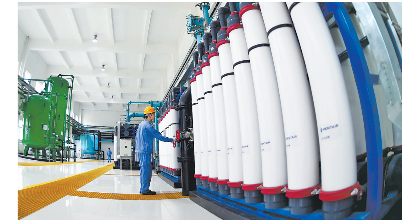
日前,京能集团涿州热电厂技术人员在化学制水车间巡检。京能集团涿州热电厂致力打造海绵式电厂,研发零水排放及智慧水网建设技术,喝的是城市再生水,吐出的废渣全部变废为宝,每年节水百余万吨。循环经济模式下,该厂成为我国北方地区第一个实现废水零排放的电厂。记者 赵永辉摄
