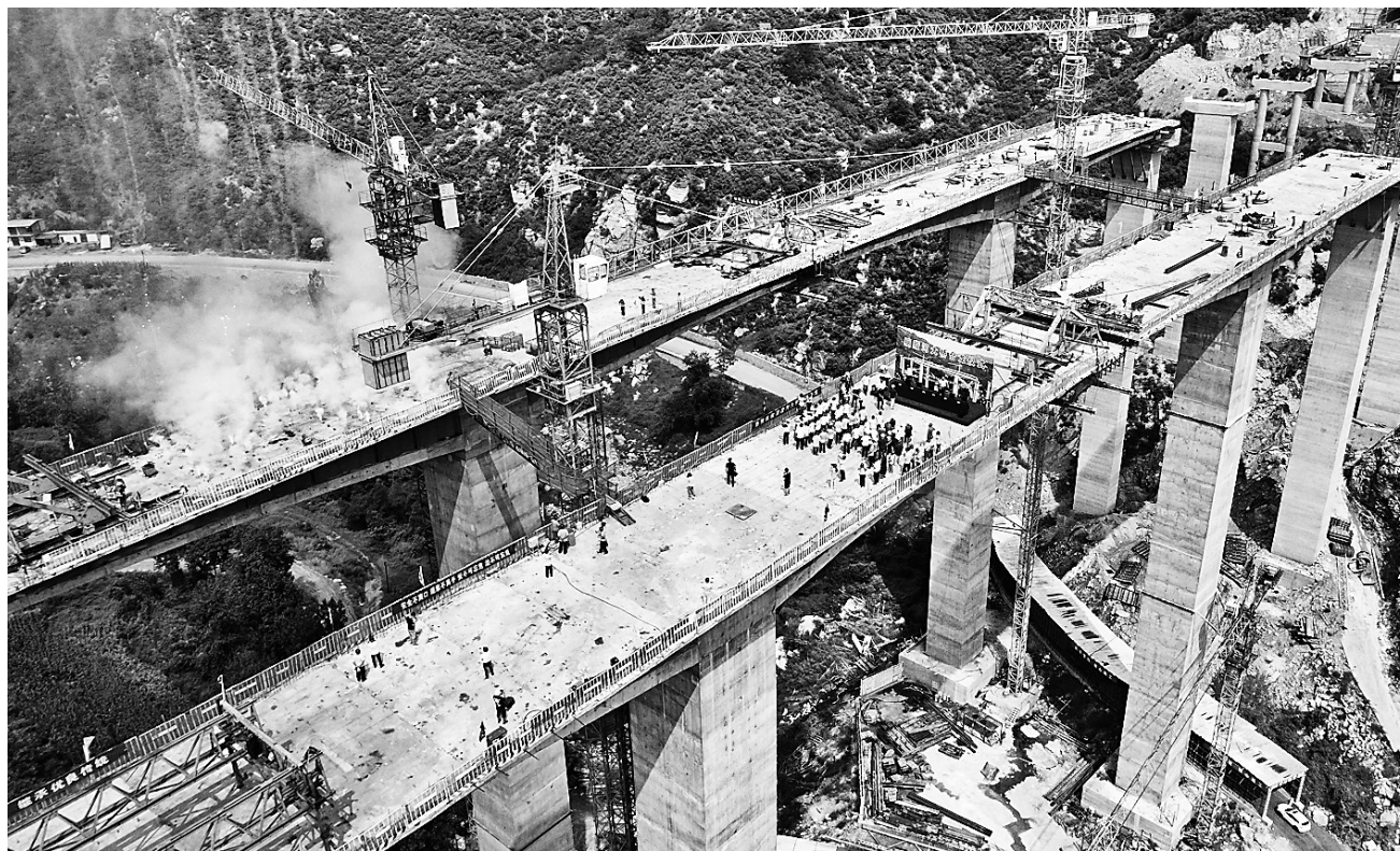
8月28日,作为太行山高速西阜保定段的重点控制性工程,胭脂河大桥主桥顺利实现合龙。此次合龙标志着太行山高速西阜保定段项目向着年底通车目标迈出了决定性一步。胭脂河大桥地处阜平县深山,属于典型的高墩大跨桥梁,是目前省内最高的波形钢腹板钢构桥。
