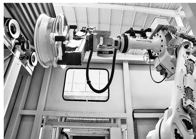
近日,中信戴卡股份有限公司总投资10亿元、年产量300万件的铝车轮六号线建成投产。该生产线通过轮毂的自动刻码设备赋予每一个轮毂独立的、唯一的身份信息,实现精准定制、精准追溯。这是轮毂自动刻码设备。 通讯员 刘文豪 张 娜摄
