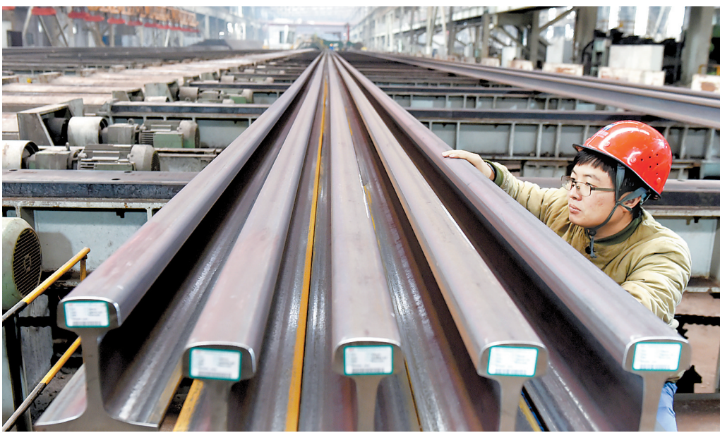
11月23日,河钢邯钢钢厂的技术人员在对刚下线的重轨进行检查。近年来,河钢邯钢着力推动产品升级,今年前10个月,重轨销售量同比增长66%,产品出口巴基斯坦、巴西、南非等多个国家和地区。记者 史晟全摄
