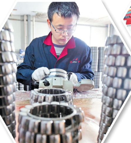
下图:临西县河北玉良轴承滚动体有限公司工人在检测E形调心滚子轴承。
