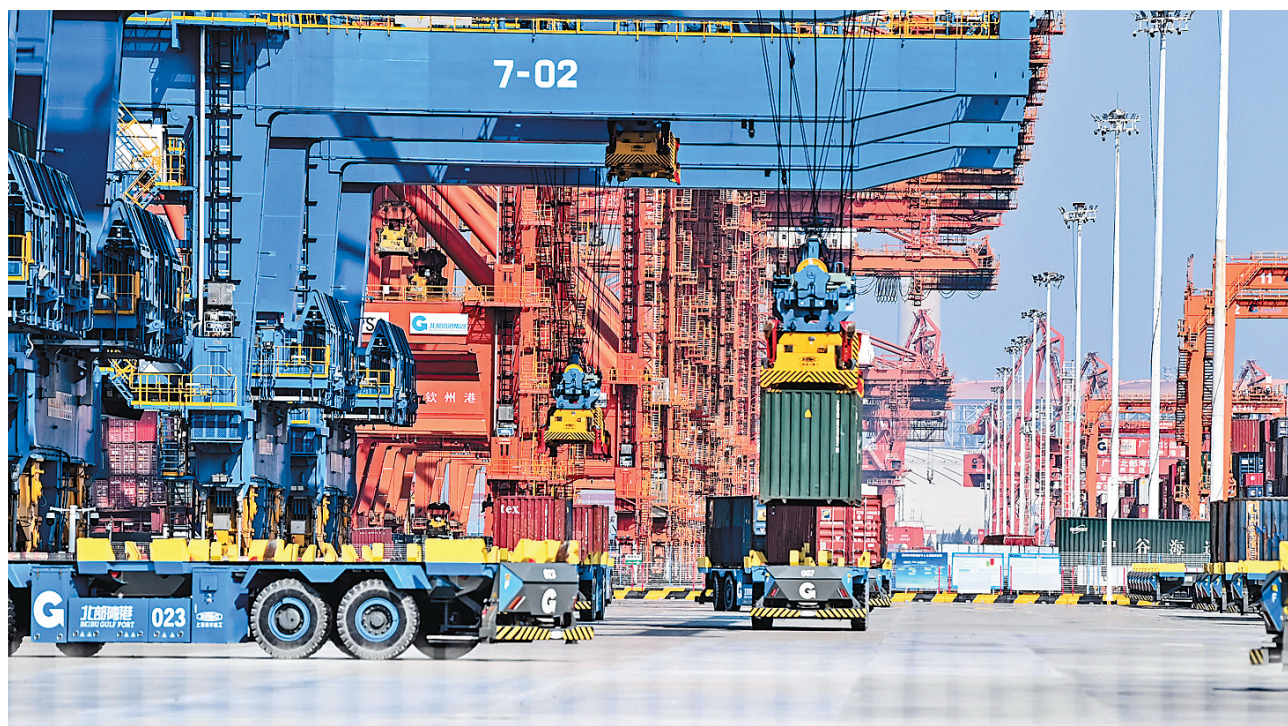
在广西钦州港自动化集装箱码头，无人驾驶车辆在转运集装箱(2023年2月25日摄)。
