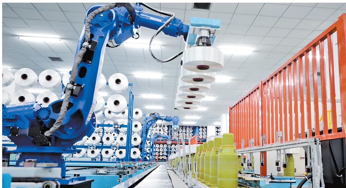
3月15日，在恒力(苏州)产业园内的高性能涤纶工业丝智能车间内，机械手臂将检验合格的丝饼放上丝车，转运至智能立体仓库。江苏省苏州工业园区是我国重要的制造业基地。近年来，当地推出多方面政策措施，促进民营企业健康发展。 新华社记者 毛俊摄
